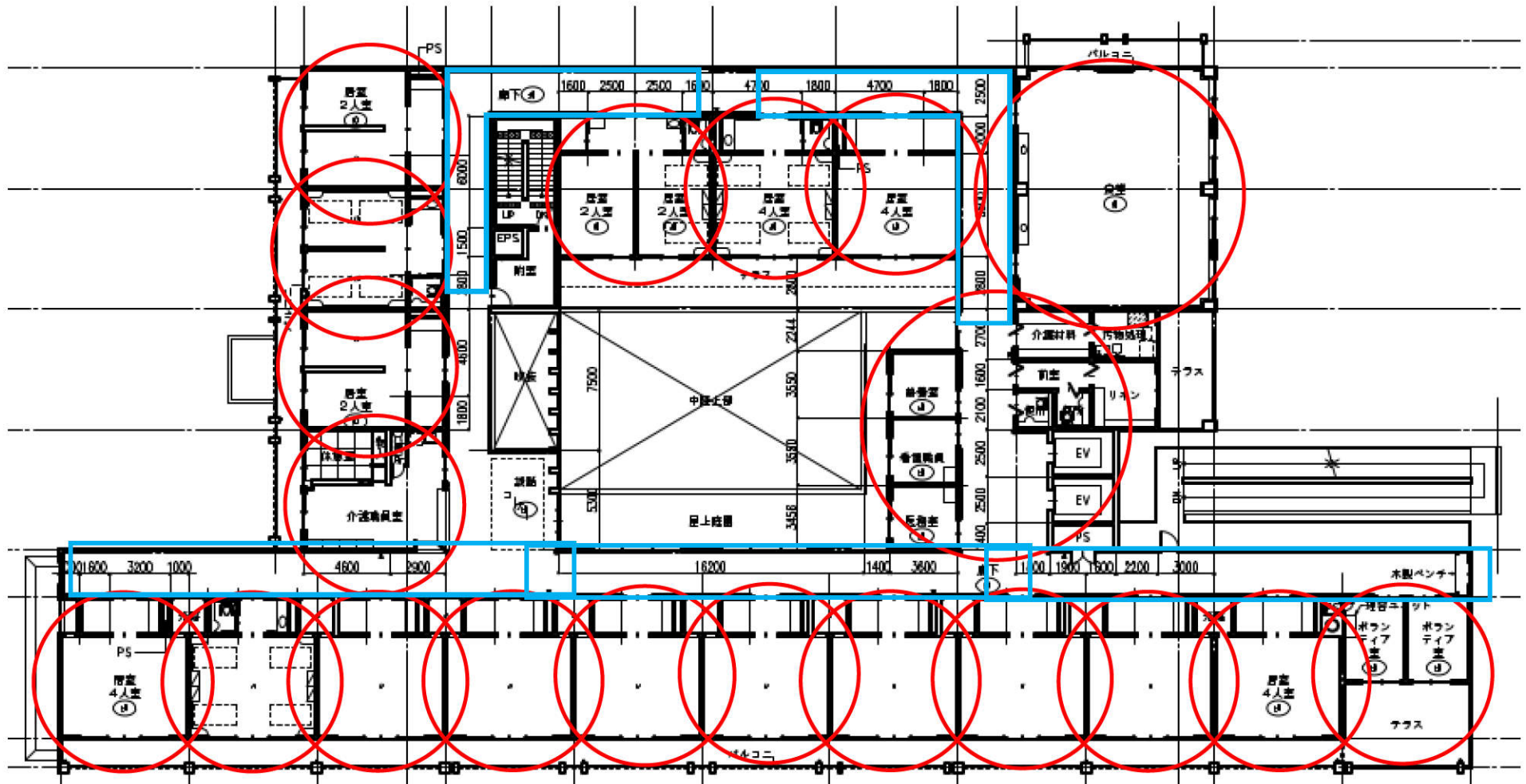
2階平面図
